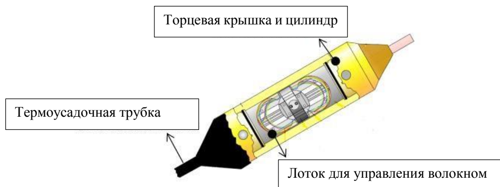
Рисунок 2-2 Схематическое изображение внутреннего блока ( 1 ) Лоток для управления оптоволоком: используется для сварки и развертывания волокон.
