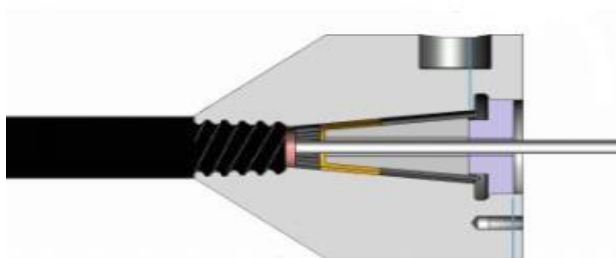
Рисунок 3-2 Принципиальная схема прессования муфты
