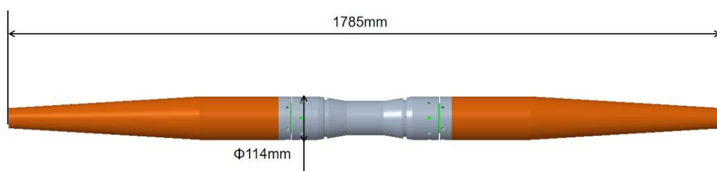
Рисунок 2-1 Корпус высокого давления BSMN-SJ-B122 SQJ и его соединительные компоненты
